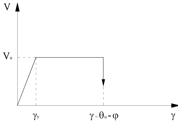
Figura 3.4 - Comportamento elasto-perfettamente plastico: taglio
