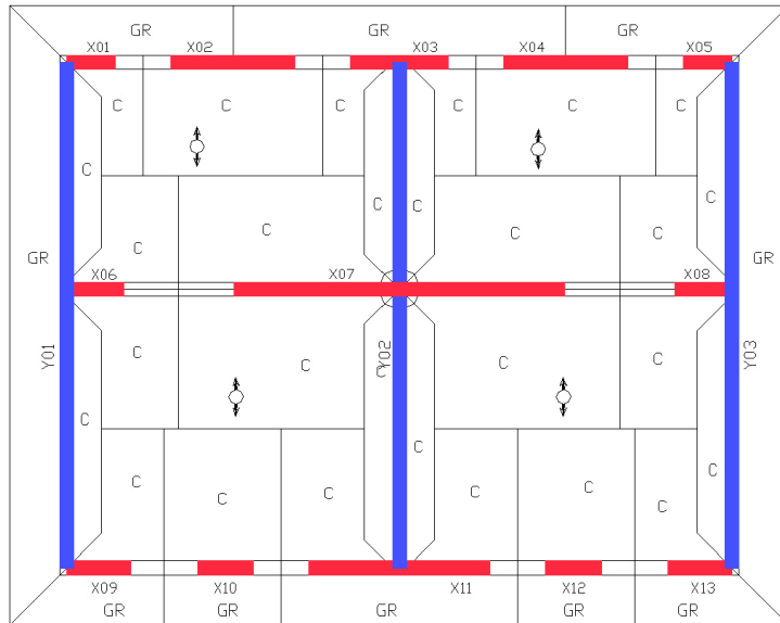
Figura 7.4 - Pianta piano sottotetto – Aree di solaio gravanti sui maschi murari del piano primo
