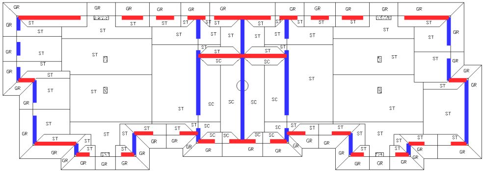
Figura 11.4 - Pianta piano sottotetto – Aree di solaio gravanti sui maschi murari del piano primo
